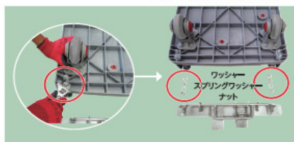
03 台車ハンドル固定部品をモンキーレンチ等で取り外す
